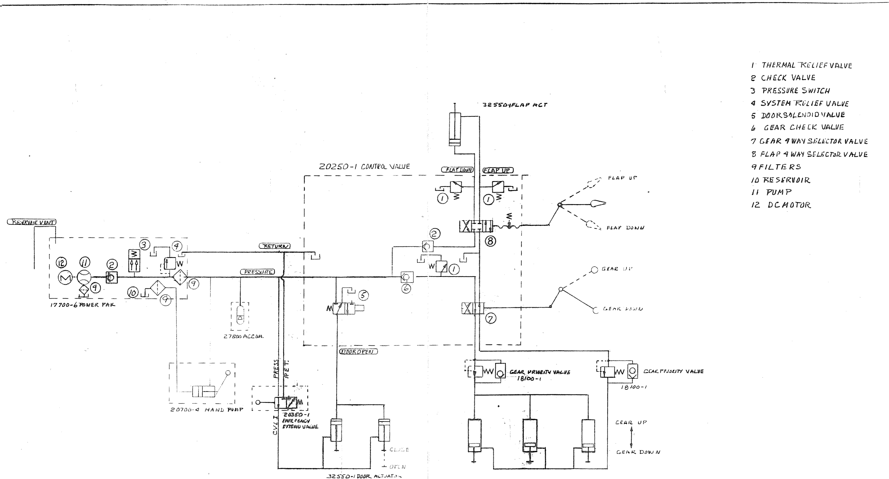
32550-1 GEAR ACTUATOR GEAR ACTUATORS
